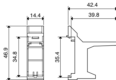
Adapter górny do montażu na szynie DIN 35 mm do serii 46.52 i 46.61
