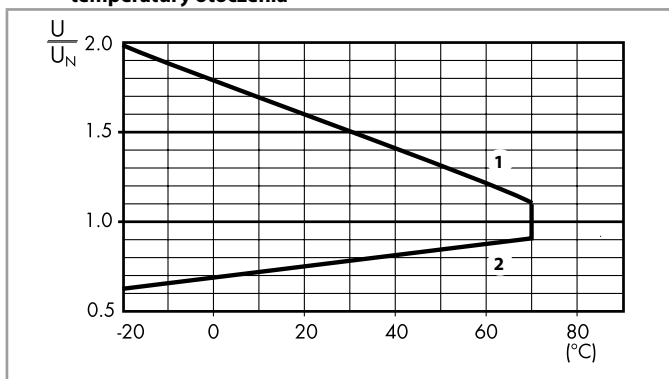
R 46 - DC Dopuszczalny zakres napięcia pracy cewki w zależności od temperatury otoczenia
