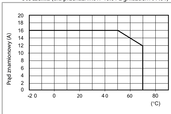
L 97 - Prąd znamionowy względem temperatury otoczenia (dla przekaźników 46.61 z gniazdem 97.01)
