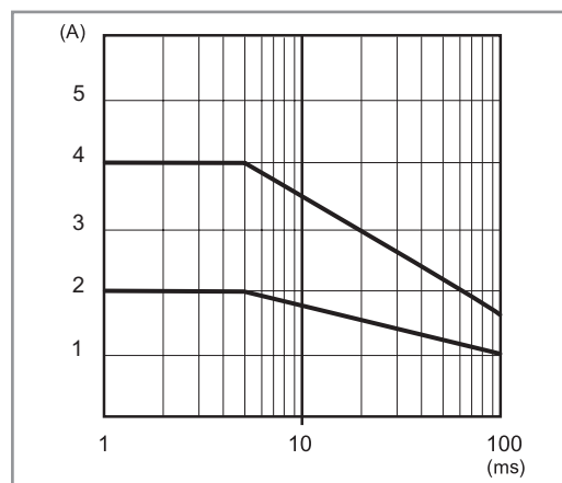
P78-1 Szczytowy prąd wyjścia w czasie (78.12)
