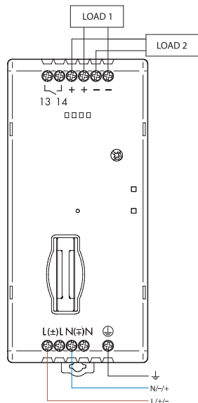
Połączenia podstawowe
