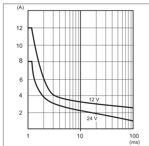
P78-2 Szczytowy prąd wyjścia w czasie (78.25)
