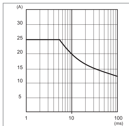
P78-11 Szczytowy prąd wyjścia w czasie (78.2E)
