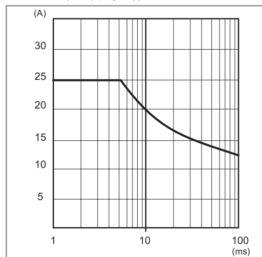
P78-10 Szczytowy prąd wyjścia w czasie (78.2A)
