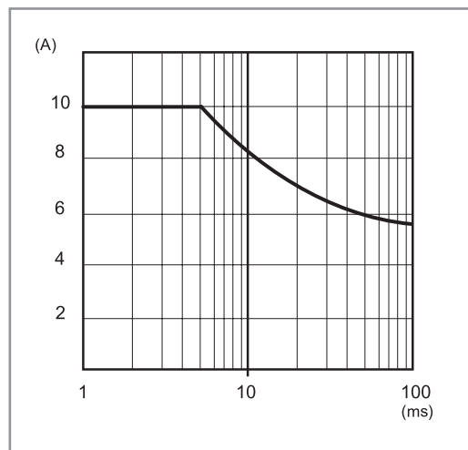
P78-8 Szczytowy prąd wyjścia w czasie (78.1B)
