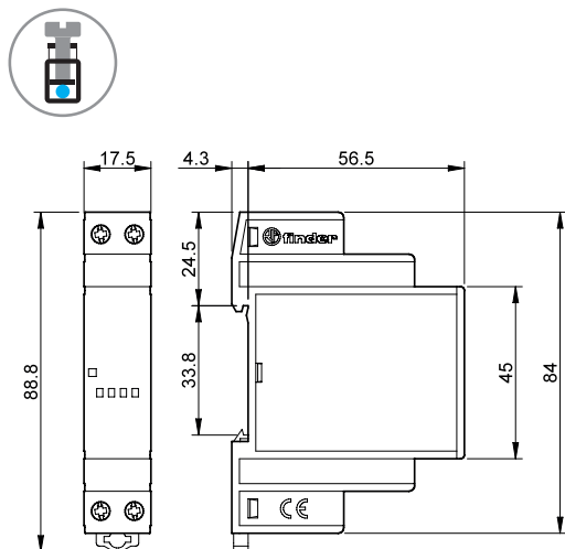
Typ 78.36 Zaciski śrubowe
