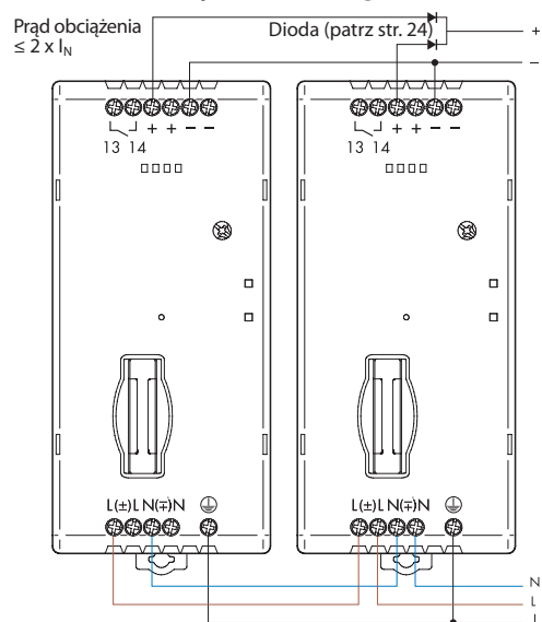
Połączenia równoległe
