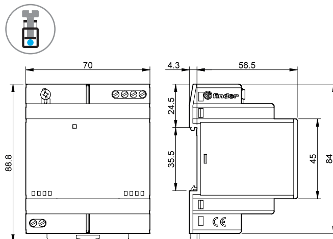
Typ 78.1B Zaciski śrubowe
