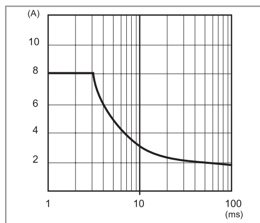
P78-3 Szczytowy prąd wyjścia w czasie (78.36)
