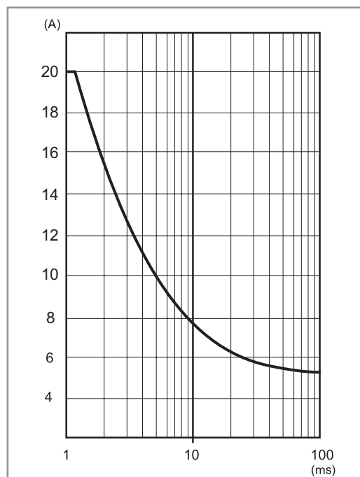
P78-9 Szczytowy prąd wyjścia w czasie (78.1D)
