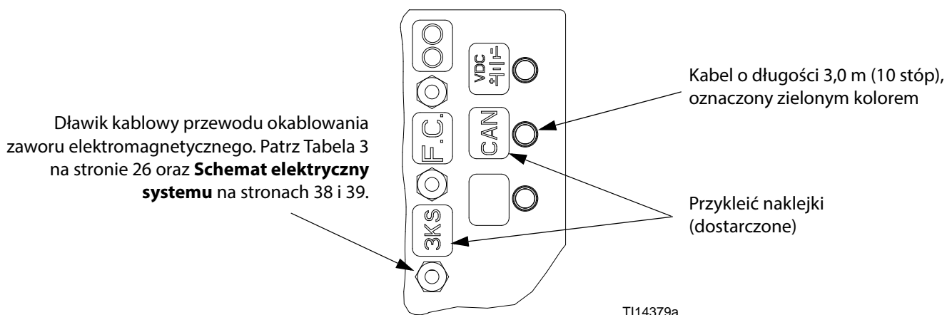
Rys. 14. Szczegółowy opis połączeń kablowych systemu ProMix 2KS
