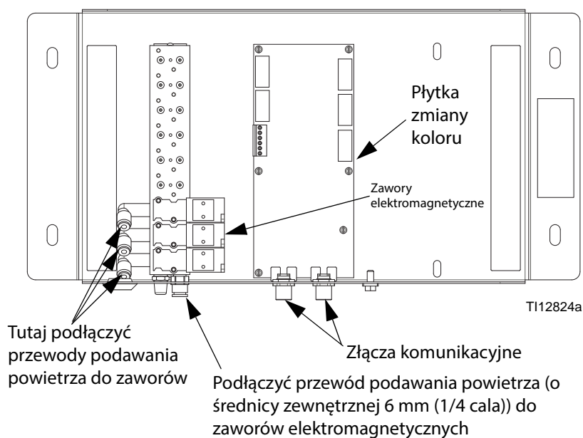
Rys. 8. Złącza hydrauliczne i pneumatyczne zaworów zmiany koloru
