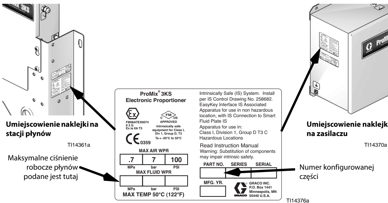
Rys. 1. Tabliczka identyfikacyjna
