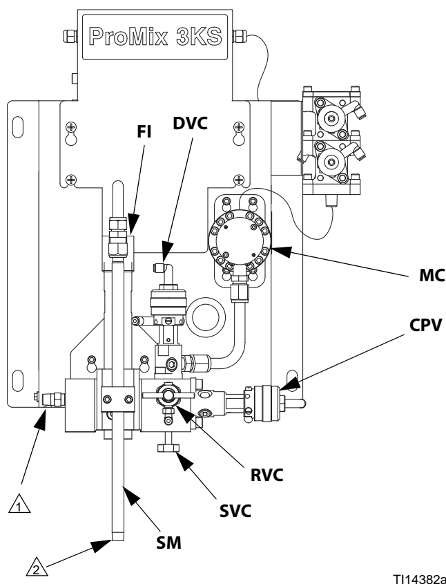
Rys. 7. Naścienna stacja płynów, dozowanie sekwencyjne
