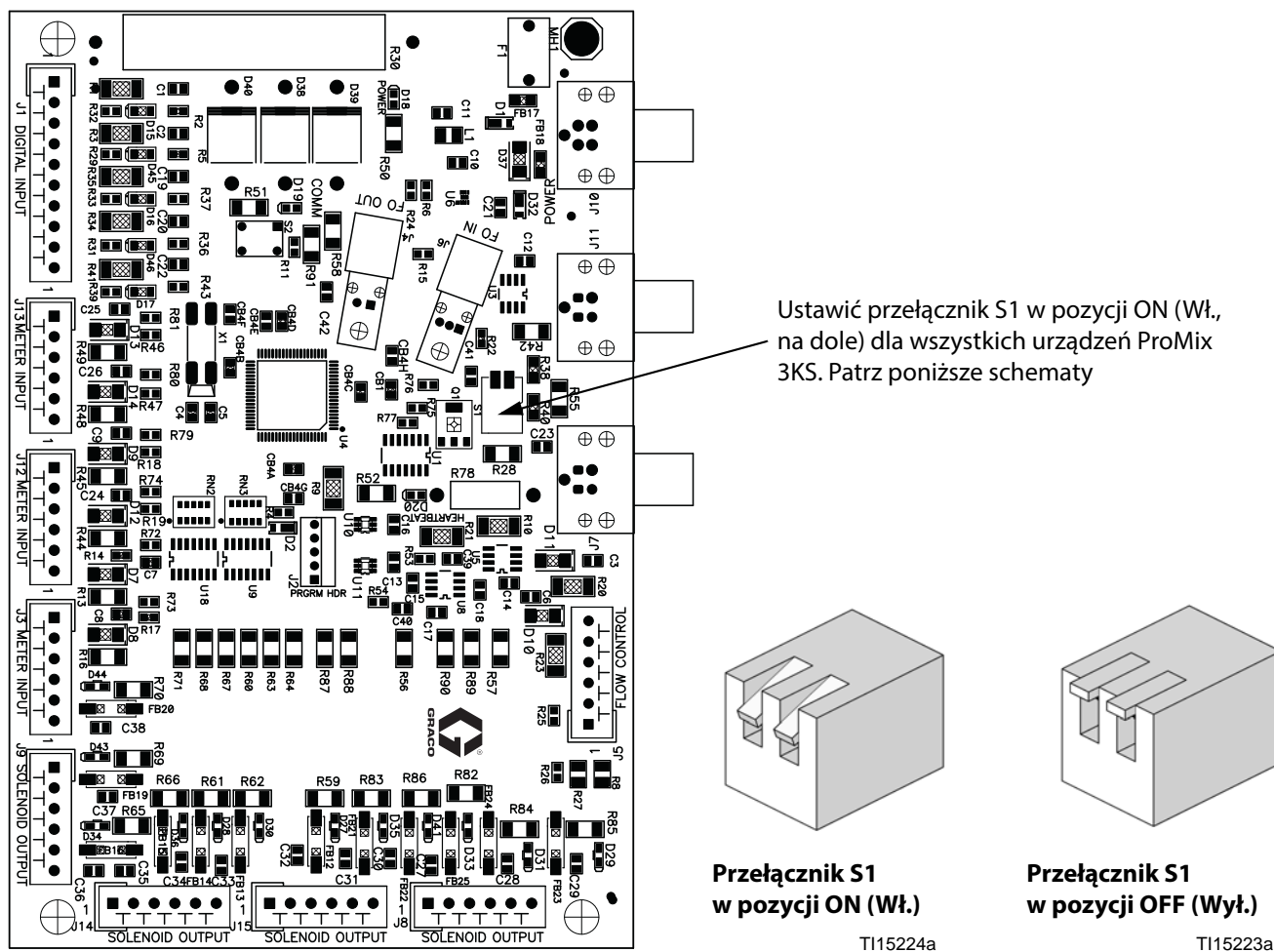
Rys. 12. 255765 Płytki sterowania stacji płynów
