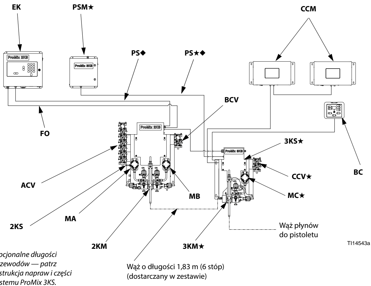
Rys. 2. Przedstawiono system ręczny z przepływomierzami G3000, sterownikiem kabiny i zmianą koloru/katalizatora/składnika C
