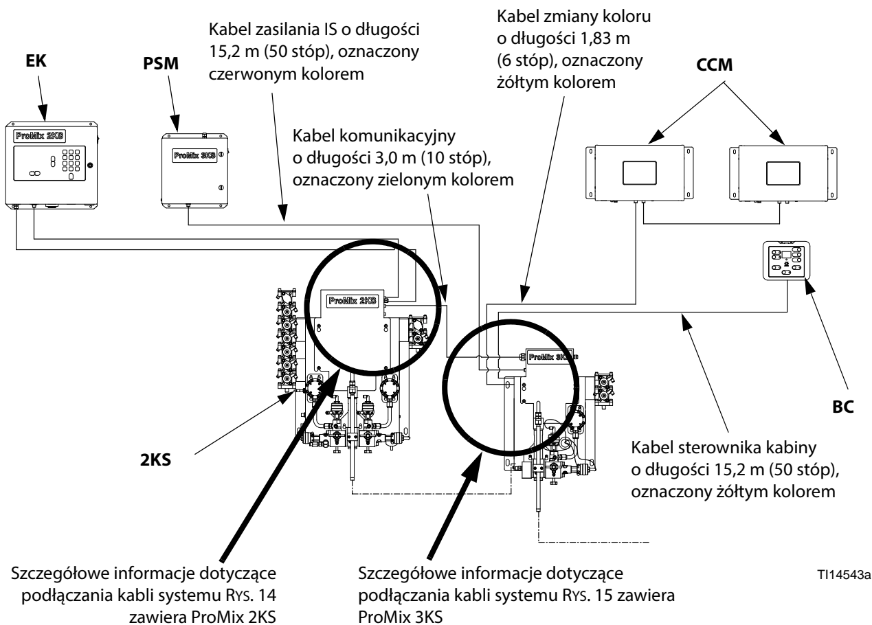
Rys. 13. Schemat okablowania systemu ProMix 3KS
