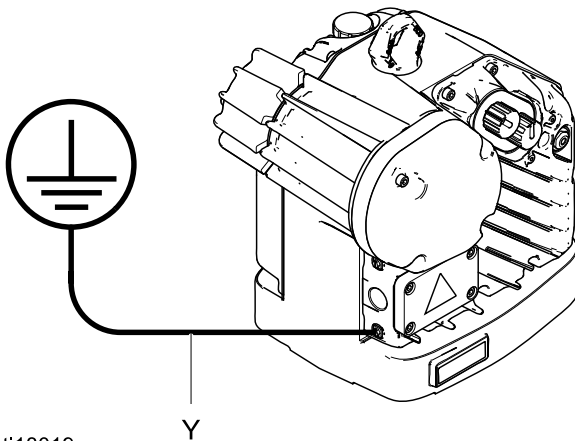
Figure 8 Przewód uziemiający
