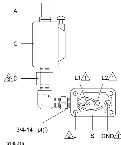
Figure 7 Podłączenie kabli zasilania
