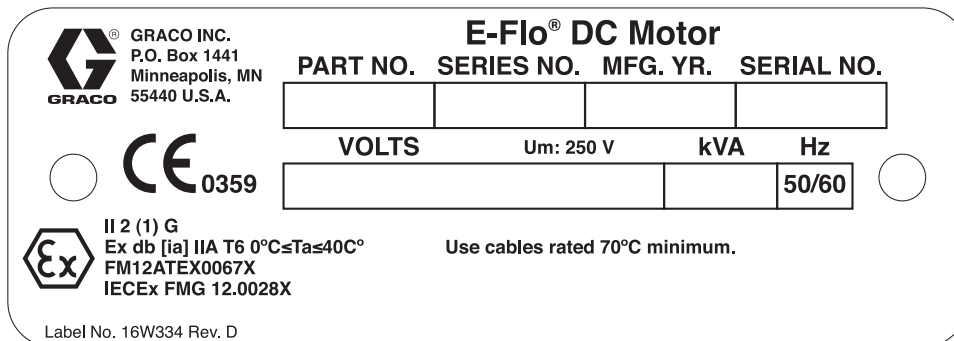
Figure 4 Zaawansowany silnik z naklejką identyfikacyjną zawierającą regionalne aprobaty
