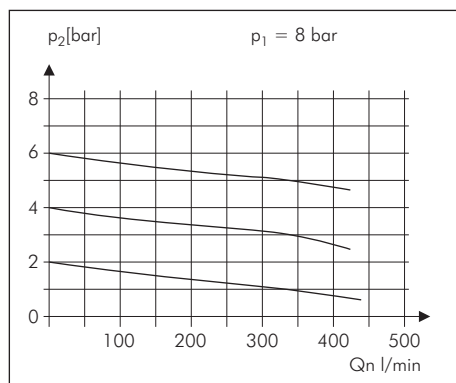
3.3. Durchflusscharakteristik
