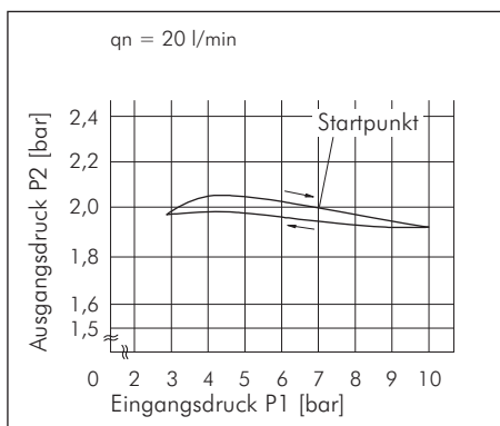
3.4. Hysterese
