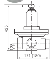
Werte in Klammern gelten für Typ Messing
