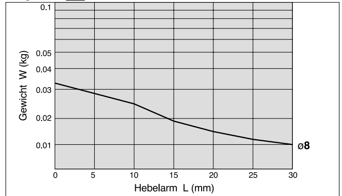
Diagramm 13 Hub: bis 30mm
