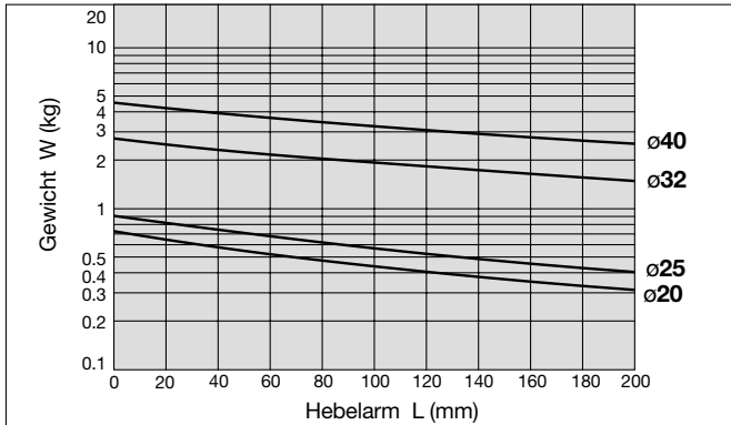
Diagramm 17 Hub: bis 200mm
