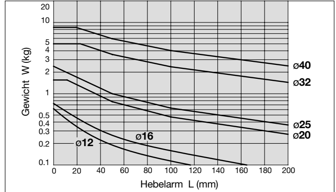
Diagramm 19 Hub: bis 100mm
