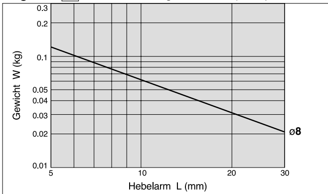
Diagramm 3 Max. Geschwindigkeit: bis 500 (mm/s)
