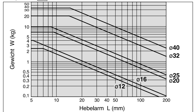
Diagramm 6 Max. Geschwindigkeit: bis 600 (mm/s)
