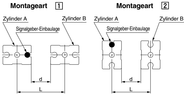
Abmessungen je Montageart
