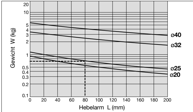
Diagramm 17 Hub: bis 200mm
