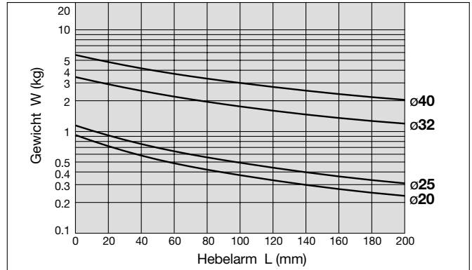
Diagramm 21 Hub: bis 200mm
