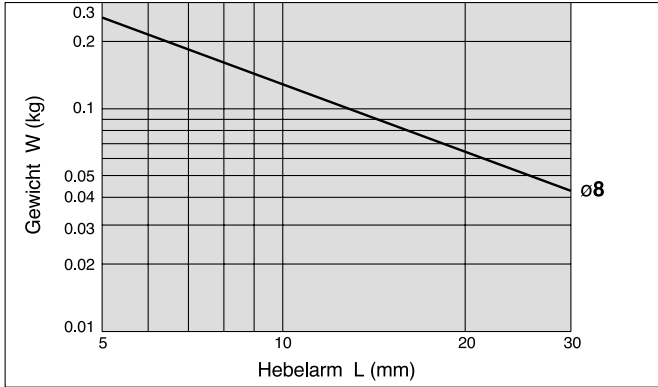
Diagramm 2 Max. Geschwindigkeit: bis 300 (mm/s)
