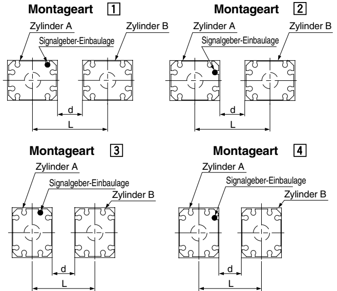
Abmessungen je Montageart
