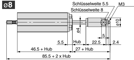
Zylinder mit Hubeinstelleinheit Ausführung mit einstellbarer Ausfahrbewegung
