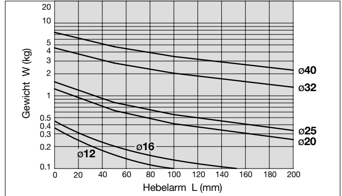
Diagramm 20 Hub: bis 150mm
