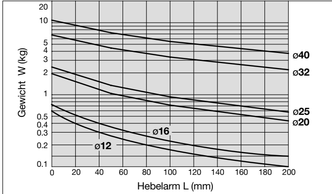
Diagramm 15 Hub: bis 100mm
