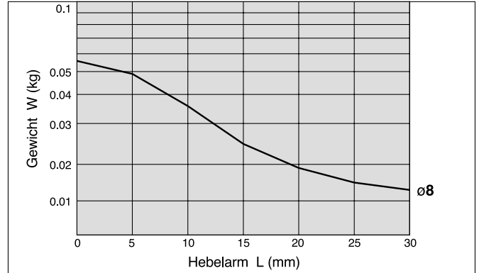
Diagramm 12 Hub: bis 20mm
