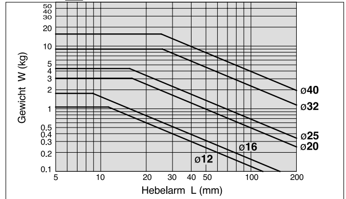
Diagramm 7 Max. Geschwindigkeit: bis 800 (mm/s)
