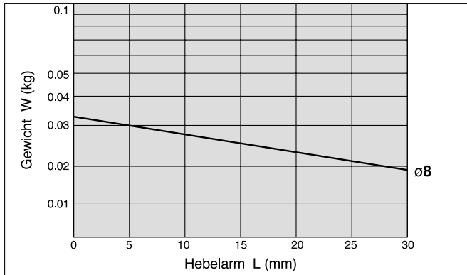
Diagramm 10 Hub: bis 30mm
