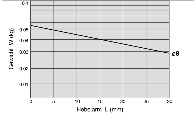
Diagramm 9 Hub: bis 20mm
