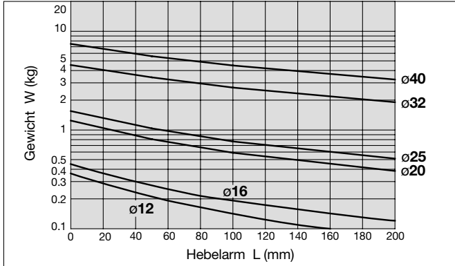
Diagramm 16 Hub: bis 150mm
