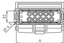
Einbauloch für Muffe
