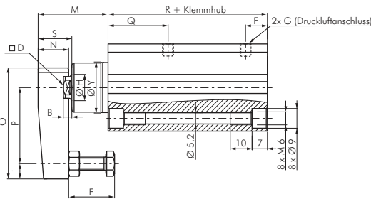
Kolben Ø 20 & 25 mm
