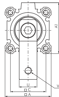
Kolben Ø 32 & 40 mm
