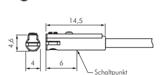
2-Leiter-Reed-Sensor
