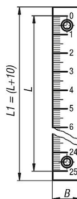
Z otworami wierconymi Położenie montażowe pionowe
